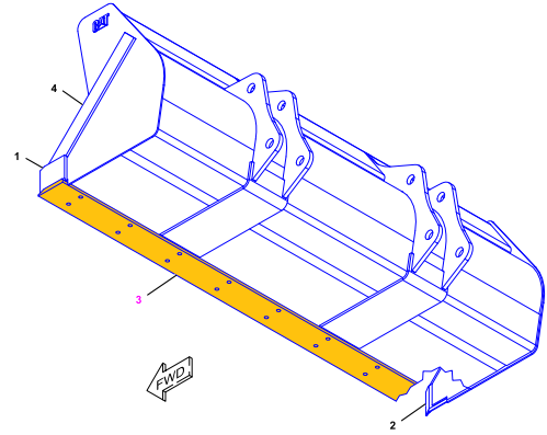
Bıçak Ağız 8 Delikli
