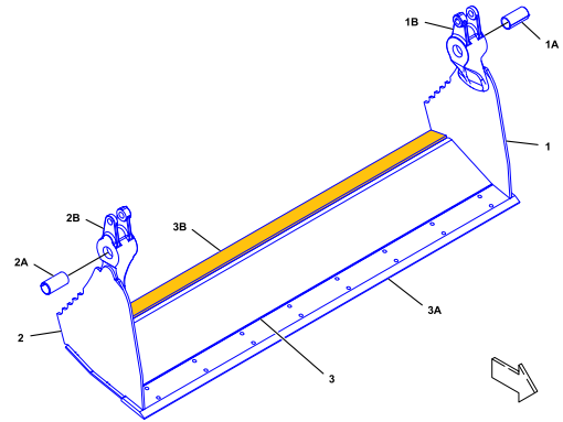
Ters Ağız
